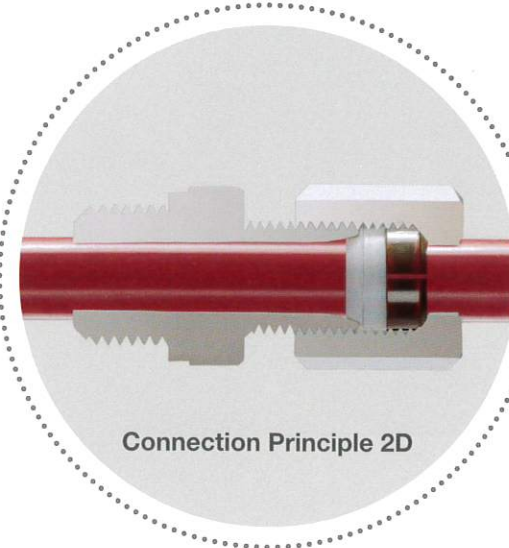
シリーズ 2D パイプ用コネクター
